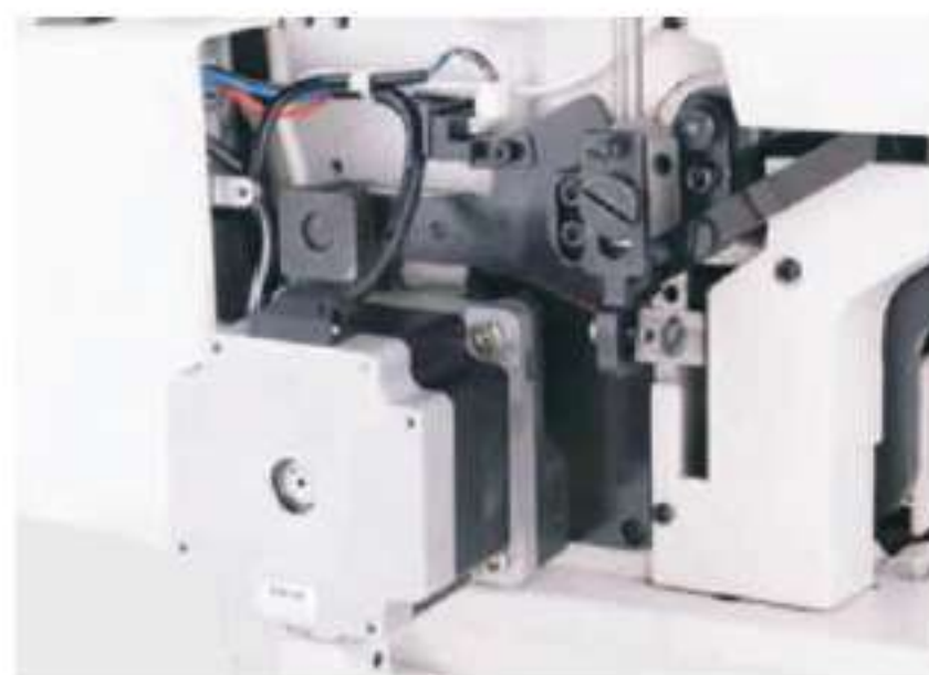
自动抬压脚，自动剪线 Auto thread trimming and presser foot lifter
